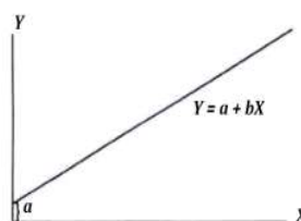
Gambar1. Ilustrasi Garis Regresi Linier
