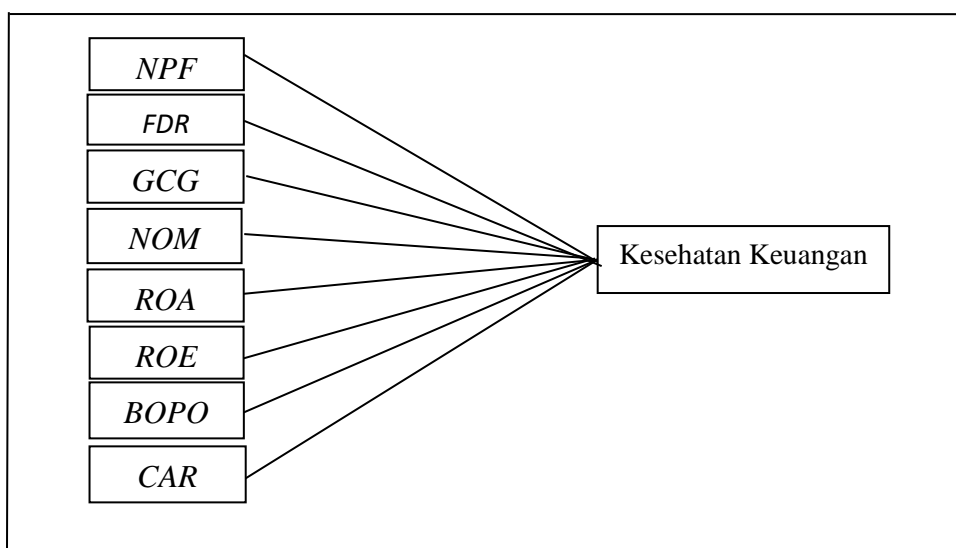
Gambar 1. Kerangka Teoritis
